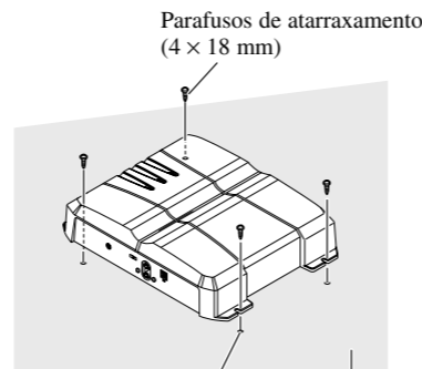
Faça um furo com um diâmetro de 2,5 mm Tapete de borracha ou chassi
